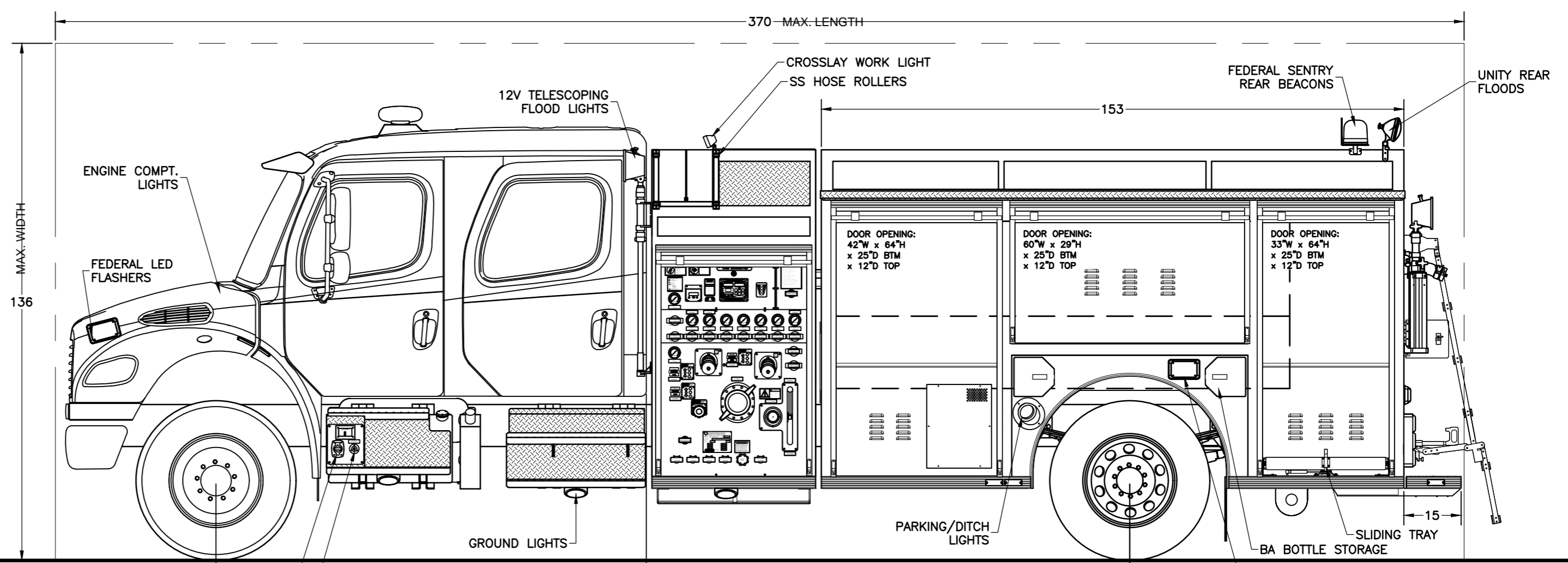
LEFT SIDE
